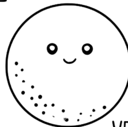
MOON
